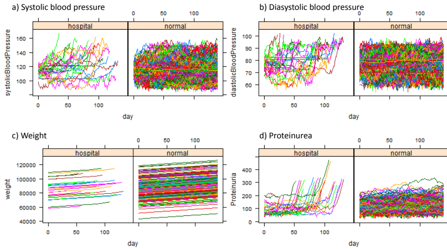
Fig. 7. Multivariate Scenario: Evaluation of variables a) - d)
